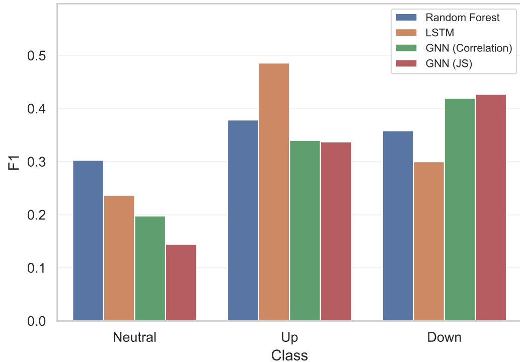
Test F1 by class
